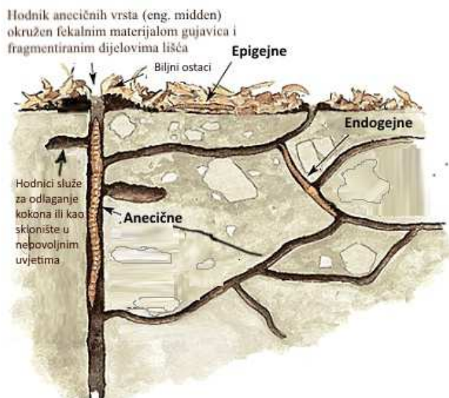
Slika 3. Tri ekološke kategorije gujavica; epigejne, endogejne i anecične (njihov položaj u profilu tla) (prilagođeno prema web 3).
