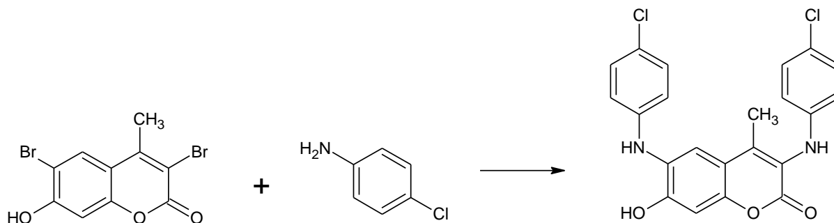
Slika 36. Priprava 3,6-bis(4-kloroanilino)-7-hidroksi-4-metil-2H-1-benzopiran-2-ona.
