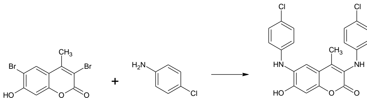
Slika 36. Priprava 3,6-bis(4-kloroanilino)-7-hidroksi-4-metil-2H-1-benzopiran-2-ona.
