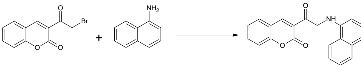
Slika 32. Priprava 3-[[1-naftalen-1-il)amino]acetil}-4a,8a-dihidro-2 H -1-benzopiran-2-ona.
