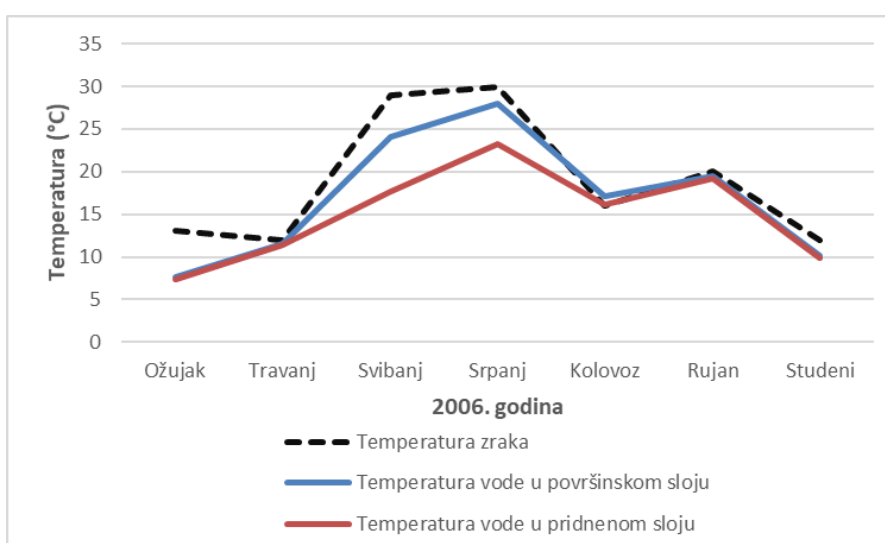
Slika 8. Promjene temperature površinskog i pridnenog sloja jezera, te temperature zraka tijekom istraživanih razdoblja 2006. godine
