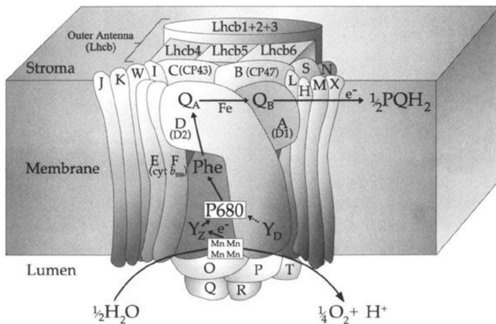
Slika 2. Fotosustav II: pregled sastava sustava i transporta elektrona. Kompleks PSII i njegov antenski sustav sastoje se od više od 20 podjedinica koje su ugrađene u tilakoidnu membranu ili povezane s njegovom lumenalnom površinom. Svjetlosna energija je zarobljena pretežno u vanjskoj anteni, koja se sastoji od proteina Lhcb1-6. Pobuđena energija se prenosi u fotokemijski aktivni centar reakcije (D1 i D2 proteini) preko CP47 i CP43, gdje se koristi za daljnje reakcije razdvajanja vode. Elektroni ekstrahirani iz vode prolaze iz lumenalno smještenog četveročlanog Mn klastera na D1-Tyr 161 (YZ), P680 + , Phe, Q A i na Q B preko nehemalne željezne skupine. Ovaj put prijenosa elektrona označen je strelicama. Protoni i molekularni kisik koji nastaju tijekom reakcije razdvajanja vode se oslobađaju u lumen. Plastokinon (PQ) vezan na Q B mjestu prihvaća dva elektrona izvedena iz vode preko elektronskog transporta lanca i dva protona iz strome prije nego što se otpušta u tilakoidnu membranu u obliku PQH 2 . Zapisivanje slova upotrijebljeno za podjedinice kompleksa jezgre odražava genetsko podrijetlo, primjerice A = produkt psbA gena (preuzeto i prilagođeno prema Hankamer, 1997).
