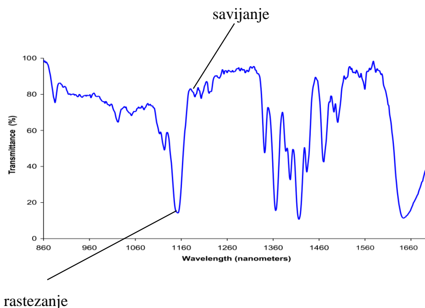
Slika 7. Infracrveni spektar
