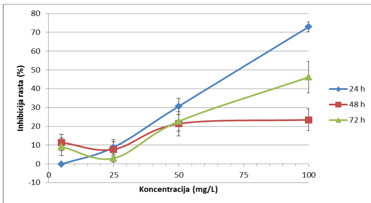
Slika 5. Postotak inhibicije rasta u kulturama M. cf. contortum 24, 48 i 72 h nakon tretmana različitim koncentracijama selenita (5, 25, 50 i 100 mg/L). Podaci su prikazani kao srednje vrijednosti \pm SD. Prosječne vrijednosti označene istim slovima (a, b, c) ne razlikuju se prema LSD testu; p < 0,05 .
