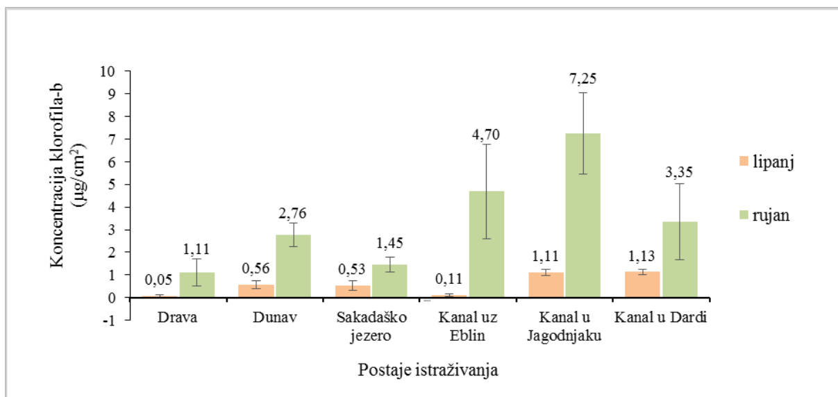
Slika 29. Koncentracija klorofila-a u sedimentu na postajama istraživanja u lipnju i rujnu 2016. godine.
