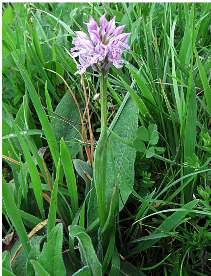
Slika 30. Habitus O. tridentata (Fotografija: M. Kovačević)
