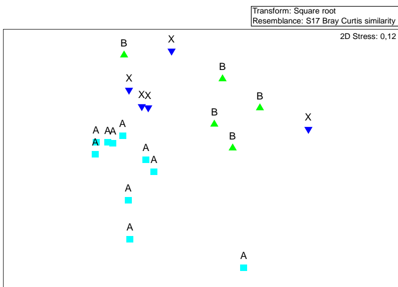
Slika 27. NMDS analiza podataka o brojnosti trzalaca prije i poslije izgradnje brane HE Lešće (oznake: ▲ B - prije brane; ■ A - poslije; ▼ x – mjesec dana nakon puštanja HE u rad)
