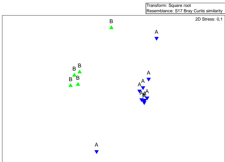
Slika 26. NMDS analiza podataka o brojnosti trzalaca prije i poslije izgradnje brane HE Lešće (oznake: ▲ B - prije brane; ▼ A – poslije)
