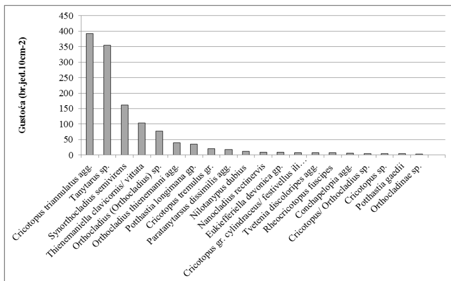
Slika 13. Prosječna gustoća (br. jed. 10 cm -2 ) eudominantnih i dominantnih vrsta/svojni trzalaca tijekom cijelog razdoblja istraživanja na postaji D7 Gojačke Dobre od 2007. do 2016. godine
