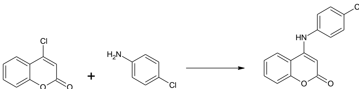
Slika 33. Priprava 4-(4-kloroanilino)-2H-1-benzopiran-2-ona.
