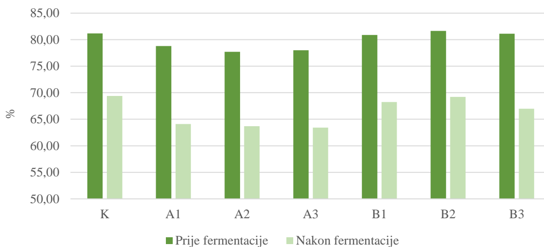
Slika 11. Prosječne vrijednosti organske tvari prije i nakon fermentacije u kontrolnoj skupini (K) te eksperimentalnim skupinama mikroalga (A1-A3) i cijanobakterija (B1-B3)
