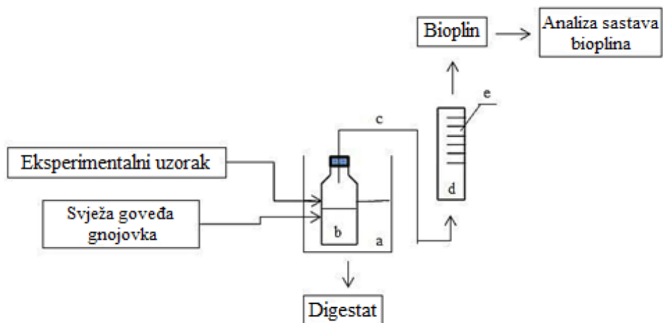
Slika 7. Shematski prikaz provedbe procesa anaerobne fermentacije: termostatska vodena kupelj (a); reaktorska boca (b); PVC cijev (c); prezasićena otopina NaCl (d); menzura za prikupljanje biolina (e) izvor: prilagođeno po Kovačić (2017)
