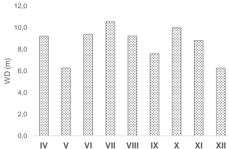
Slika 5. Mjesečne vrijednosti dubine rijeke Dunav za vrijeme uzorkovanja u razdoblju od travnja do prosinca 2011.
