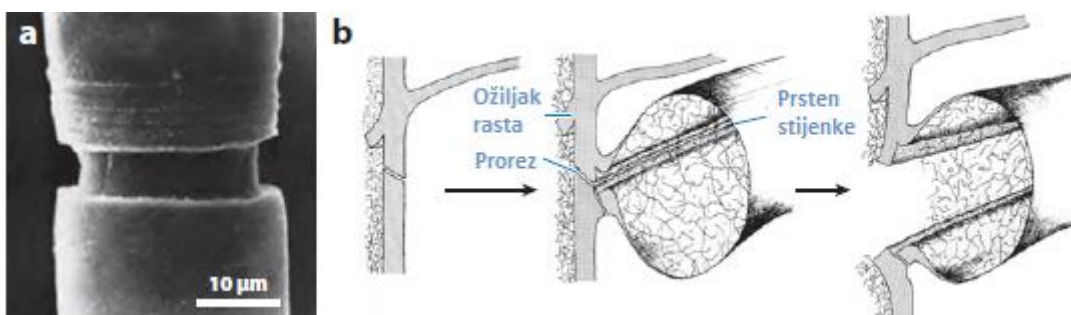
Slika 1. Mehaniizam ekspanzije stanica algi iz roda Oedogonium a) ekspanzirajući unutrašnji prsten stijenke; b) razvoj prstena stijenke i rana faza ekspanzije. Prsten stijenke razvija se unutar stanice na razini proreza u nosivoj stijenci. Fraktura vanjske stijenke uz prorez stavlja unutrašnji prsten stijenke pod opterećenje, što omogućuje naglu elongaciju stanice (prilagođeno prema Pickett-Heaps, 1975).
