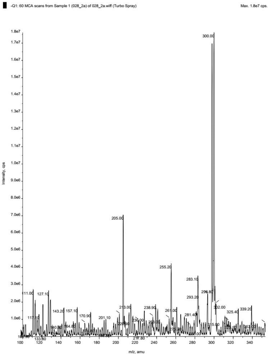
Slika 18: Maseni spektar (5Z)-5-(3-brombenziliden)-2-tio-1,3-tiazolidin-4-ona
